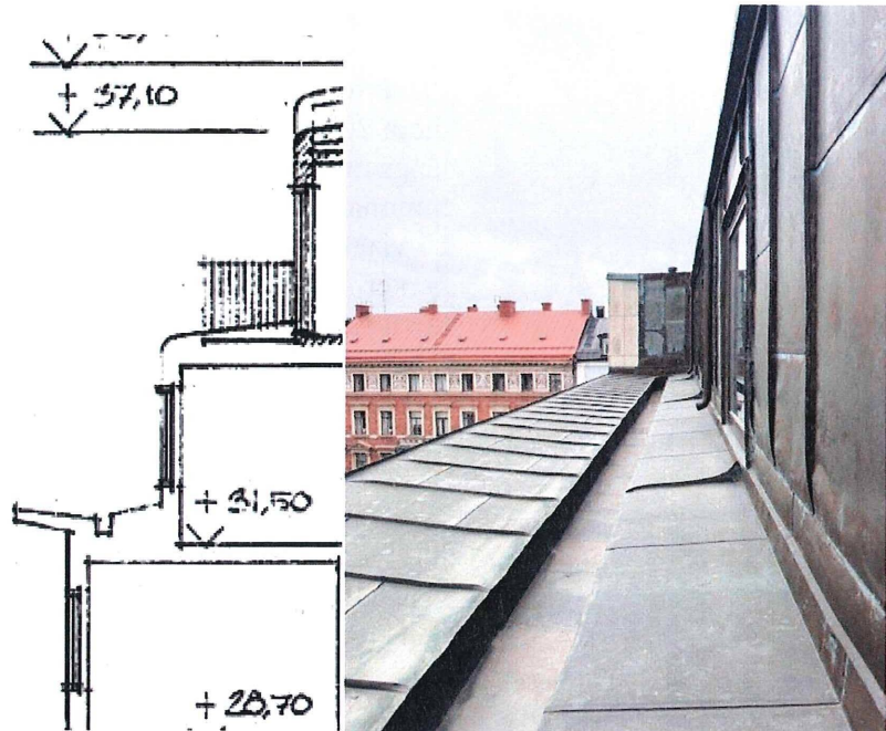
Bilden till vänster visar sektion på ursprunglig utstickande takfotsgesims och det karaktäristiska rundade taket. Bilden till höger visar takfotsgesimsens bruna kopparkulör och utförande sett från plan 7 mot Nybrogatan. Bild: Nyréns och Stadsbyggnadskontoret.
