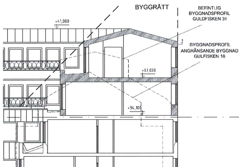
Bilden visar Guldfisken 31 i fonden med dess beviljade tillbyggnad. I sektion redovisas dess tidigare höjd samt relation till Guldfisken 18. Bild: Stadsbyggnadskontoret.
