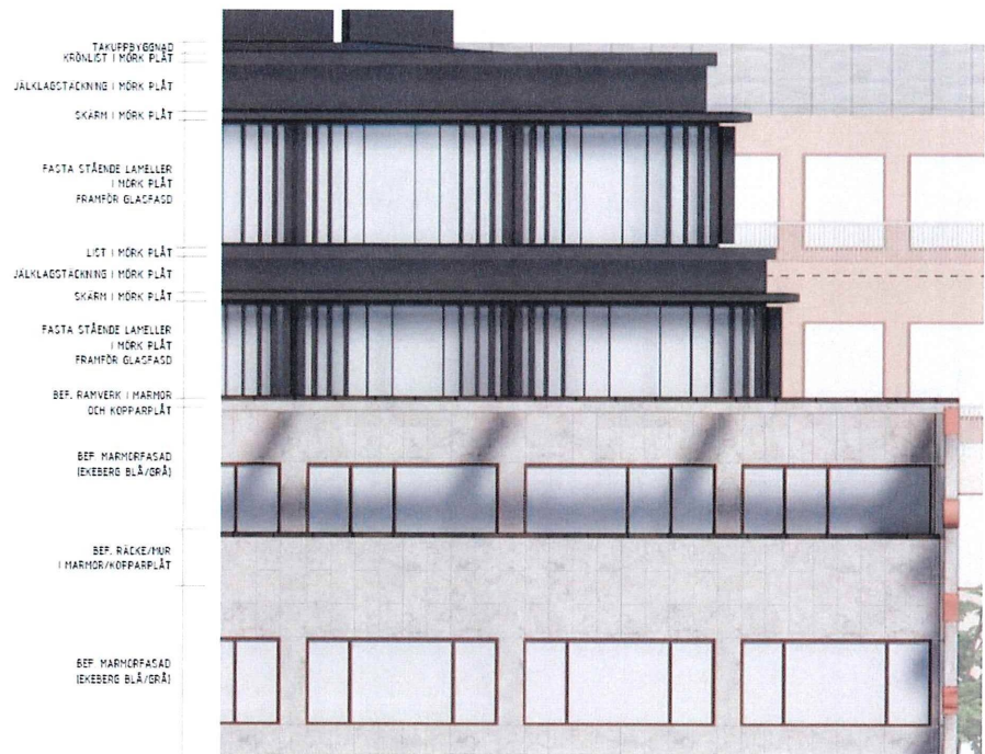
Bilden visar fasadutsnitt med föreslagen påbyggnad med namngivna detaljer, fasad mot öster. I förgrunden visas Guldfisken 31 med möjlig påbyggnad, streckad linje befintlig höjd. Bild: Nyréns
